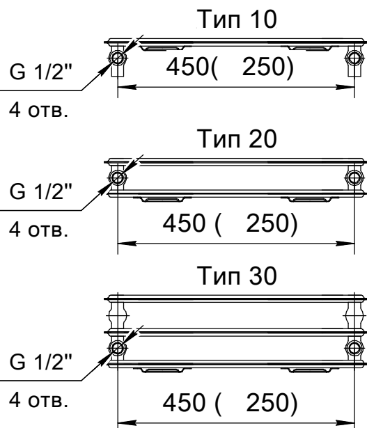
Рисунок 2 - Основные монтажные размеры для подключения.
